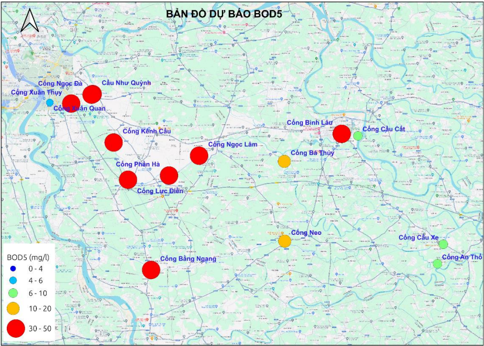
Hình 5: Bản đồ dự báo BOD 5
