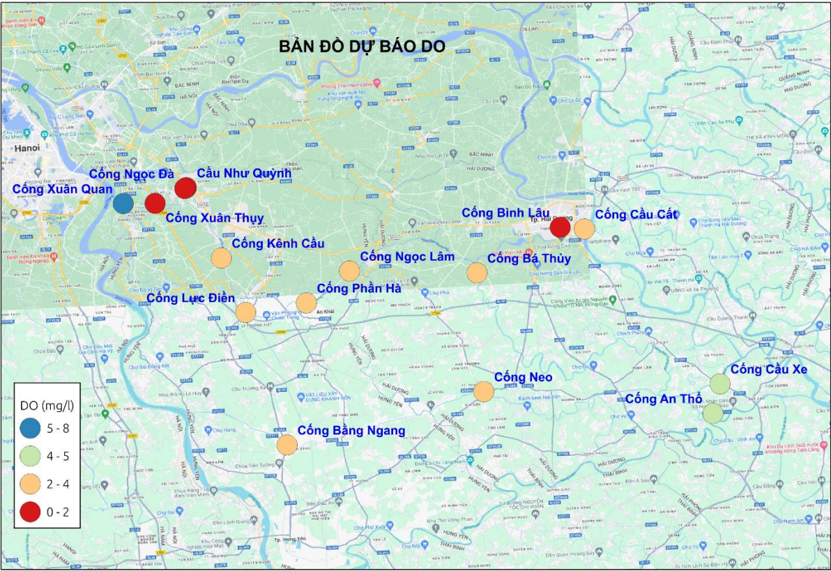
Hình 3: Bản đồ dự báo DO
