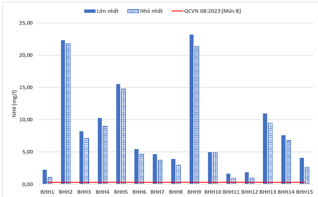
Hình 6: Biểu đồ so sánh kết quả dự báo \text{NH}_4^+
