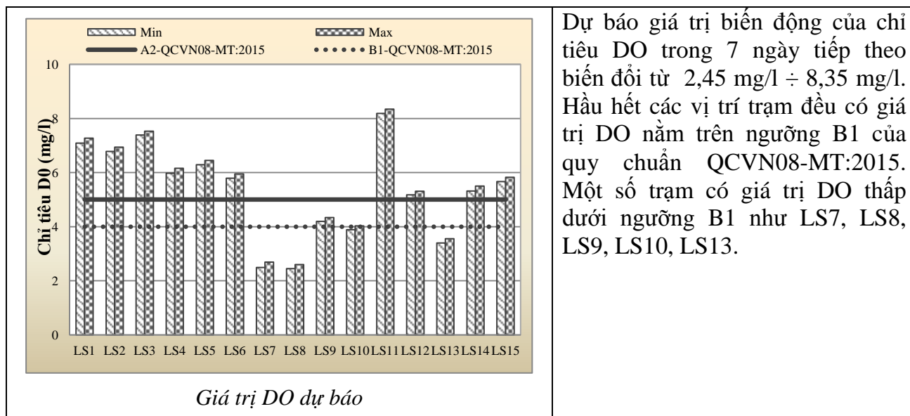
Bảng 1. Kết quả dự báo thông số DO các trạm đến ngày 13/03/2018
