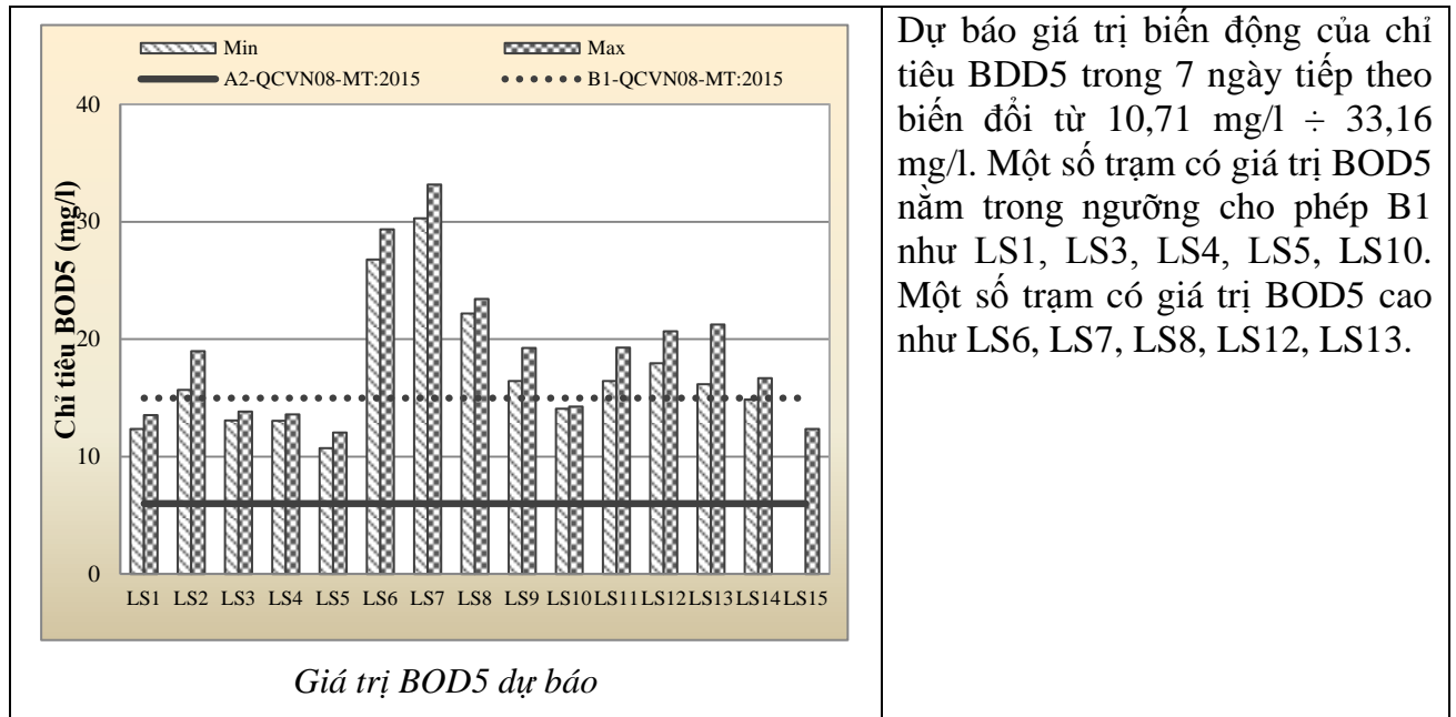
Bảng 2. Kết quả dự báo thông số BOD5 các trạm đến ngày 13/03/2018
